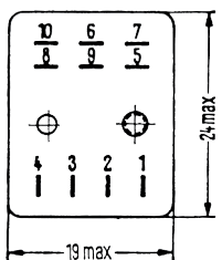
V23162-A0xx, size I type
